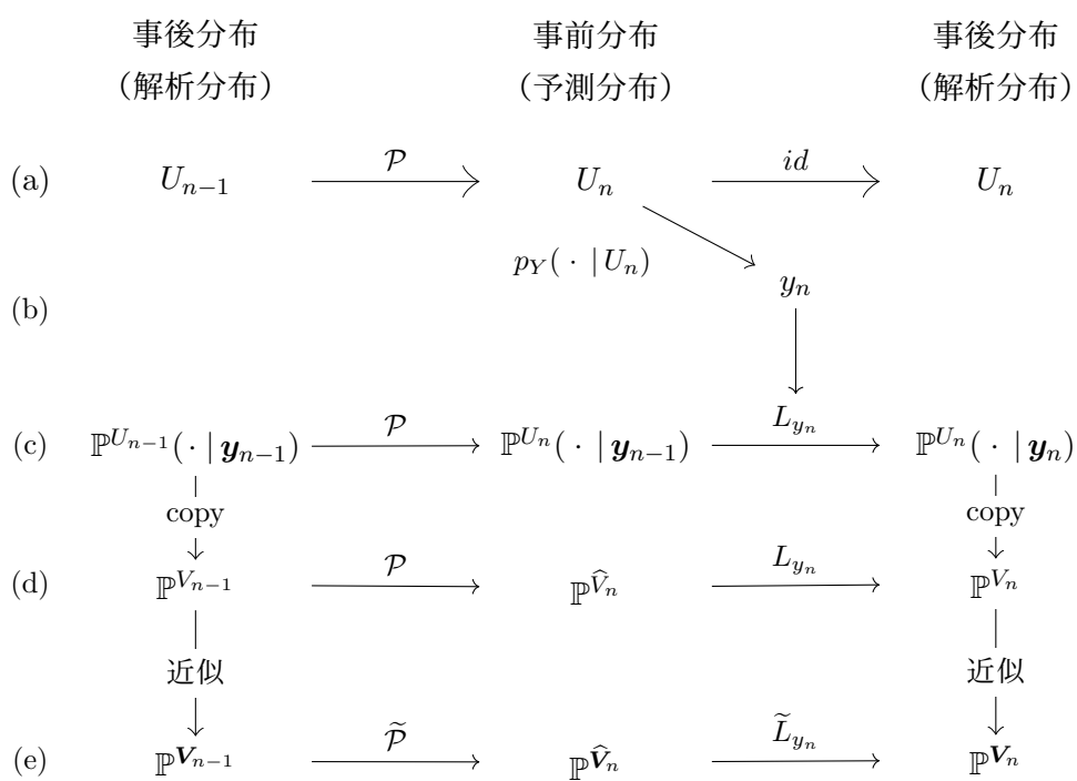
図 2: フィルタリング問題における階層. 階層は (a) モデルダイナミクス, (b) 観測, (c) 条件付き分布, (d) 厳密なフィルタ分布, 及び (e) 近似されたフィルタ分布である.
