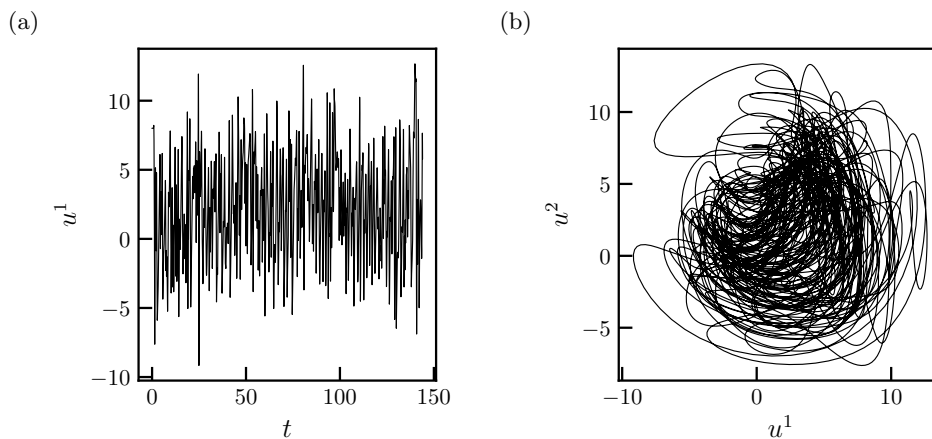
図 5: L96 方程式 (5.6) の解 ((J, f) = (40, 8)) .
